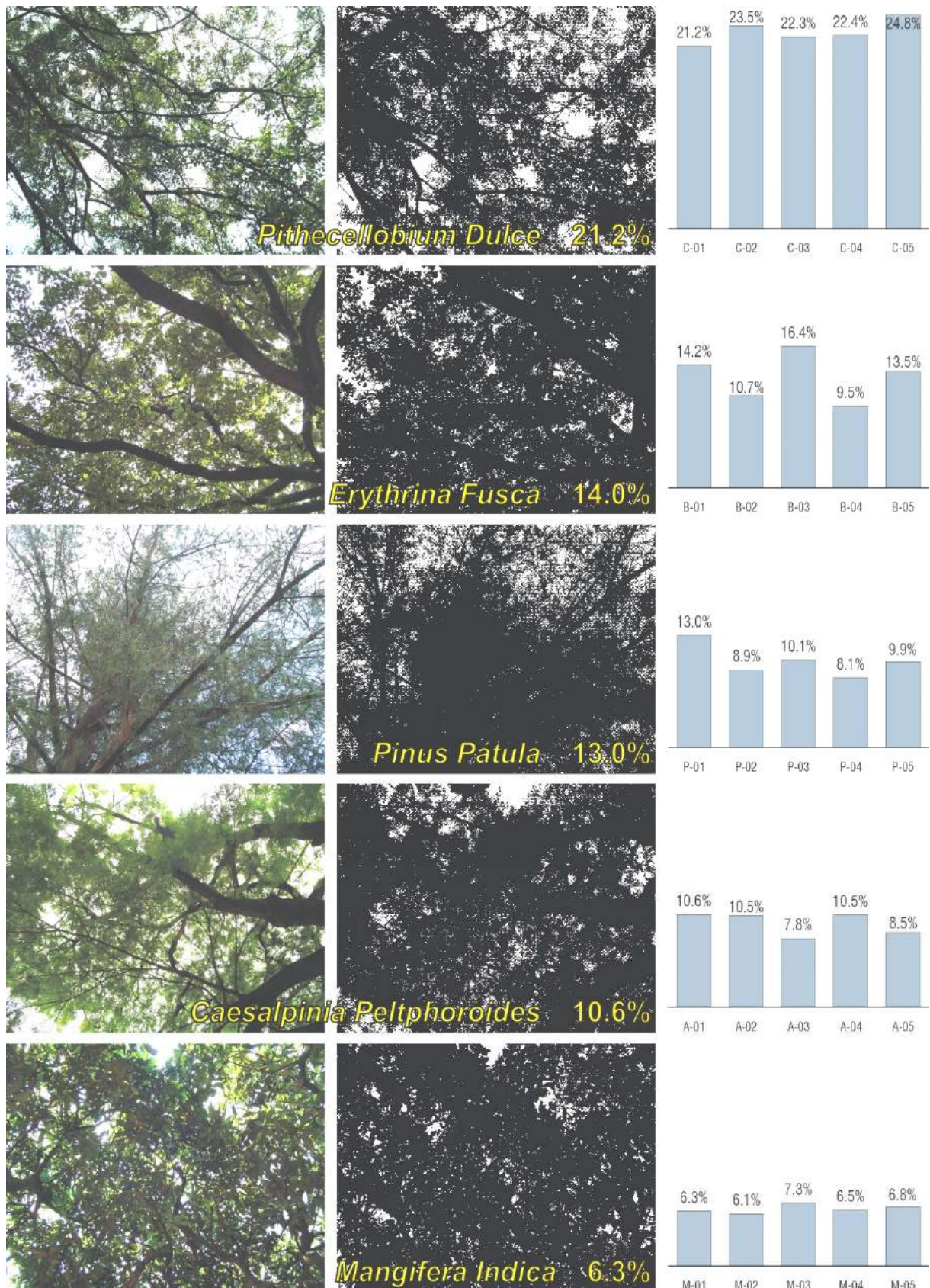
Figura 5 –Transparencia cenital del follaje de cinco árboles de uso típico en los proyectos de silvicultura urbana en Medellín. A la izquierda, fotografías verticales de abajo hacia arriba de árboles adultos tomadas en un día nublado. En el medio, procesamiento de las imágenes para calcular la porción de la imagen que corresponde al cielo visto a través del follaje, las ramas y las semillas. A la derecha, parte de los resultados numéricos obtenidos al procesar las fotografías de 20 ejemplares de cada una de las especies en estudio. Es claro que cada ejemplar tiene una sombra única, no obstante, existe una clara relación entre especie y Factor de Transparencia. Esta metodología permitió caracterizar cada especie no sólo por su Huella de Sombra, sino también por la densidad de la misma. Fotografías con diferentes ángulos de inclinación permitirán en futuros proyectos estudiar la variación de la densidad de sombra en función del ángulo de altura solar.
