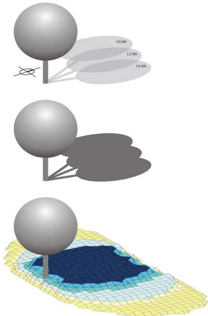
Figura 2 – Superposición de las sombras que a diferentes horas del día durante los meses de noviembre a enero proyecta un árbol de copa esférica ubicado en la ciudad de Medellín. Los tonos más oscuros corresponden a los sectores que permanecen sombreados con una mayor frecuencia.
